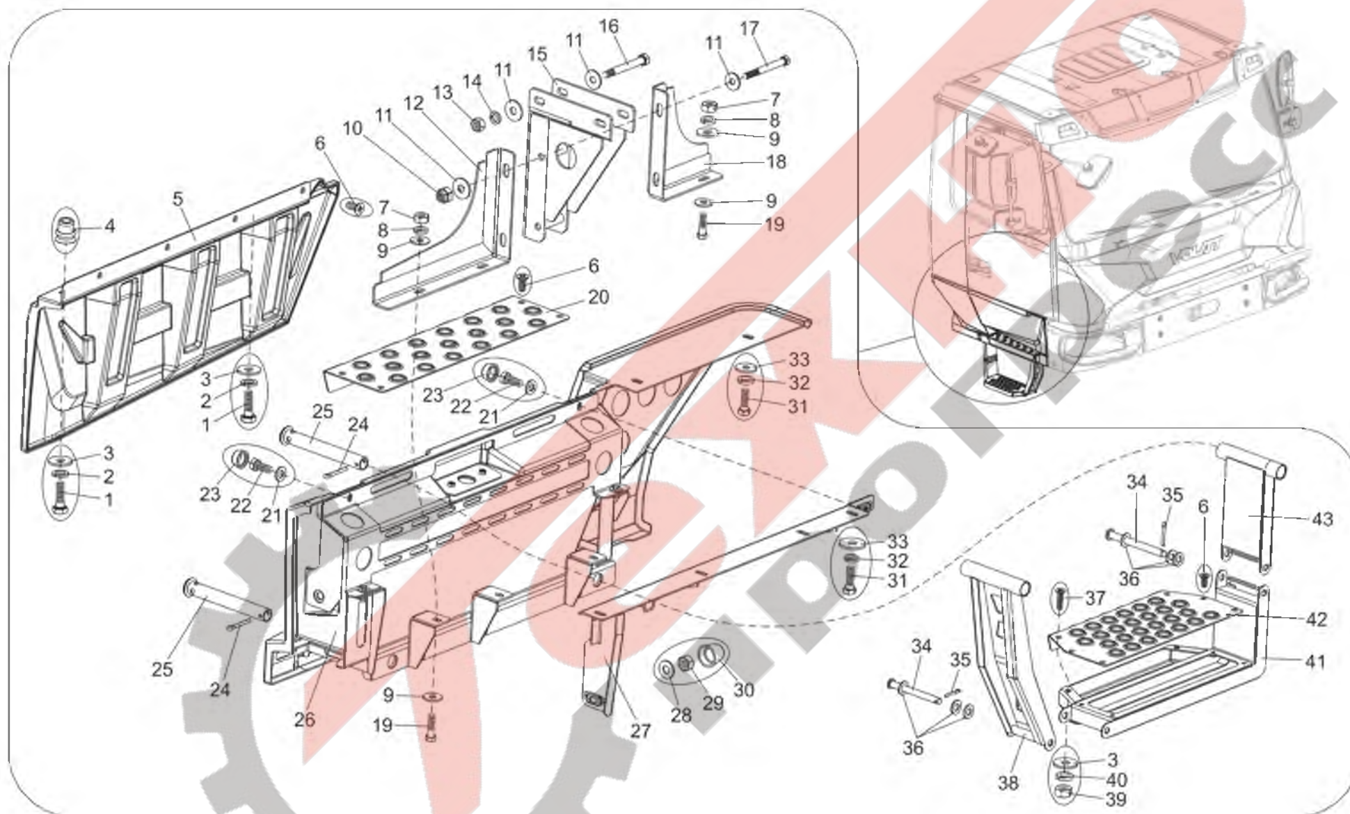
Рис. / Fig. 84.5 Установка подножек. Правая сторона / Installation of step plates. Right side 750002-8400008
