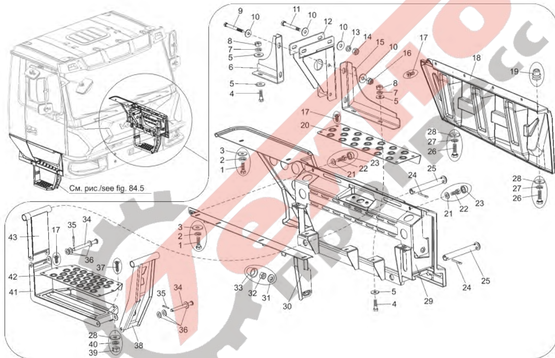
Рис. / Fig. 84.4 Установка подножек. Левая сторона / Installation of step plates. Left-hand side 750002-8400008
